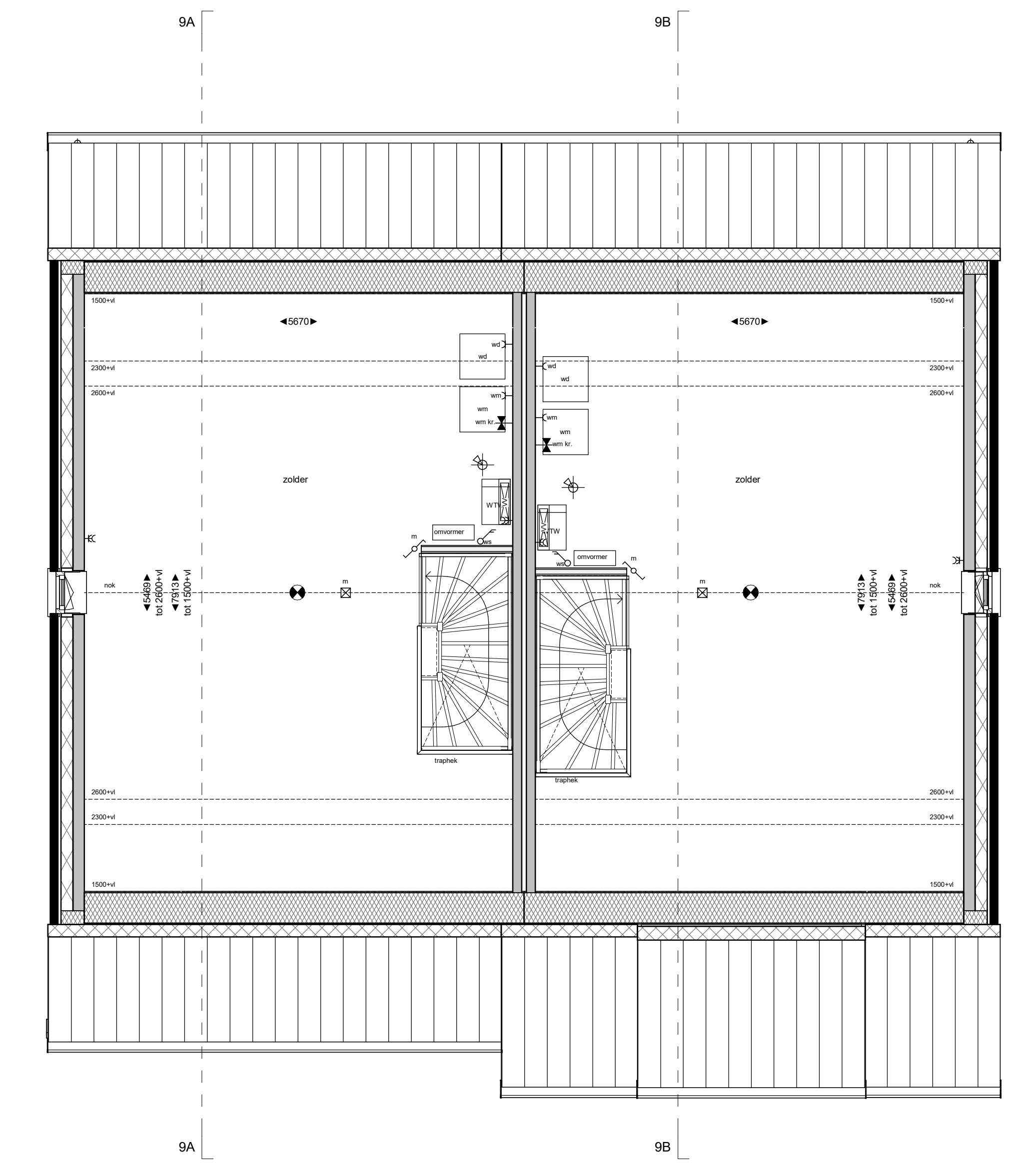
tweede verdieping
