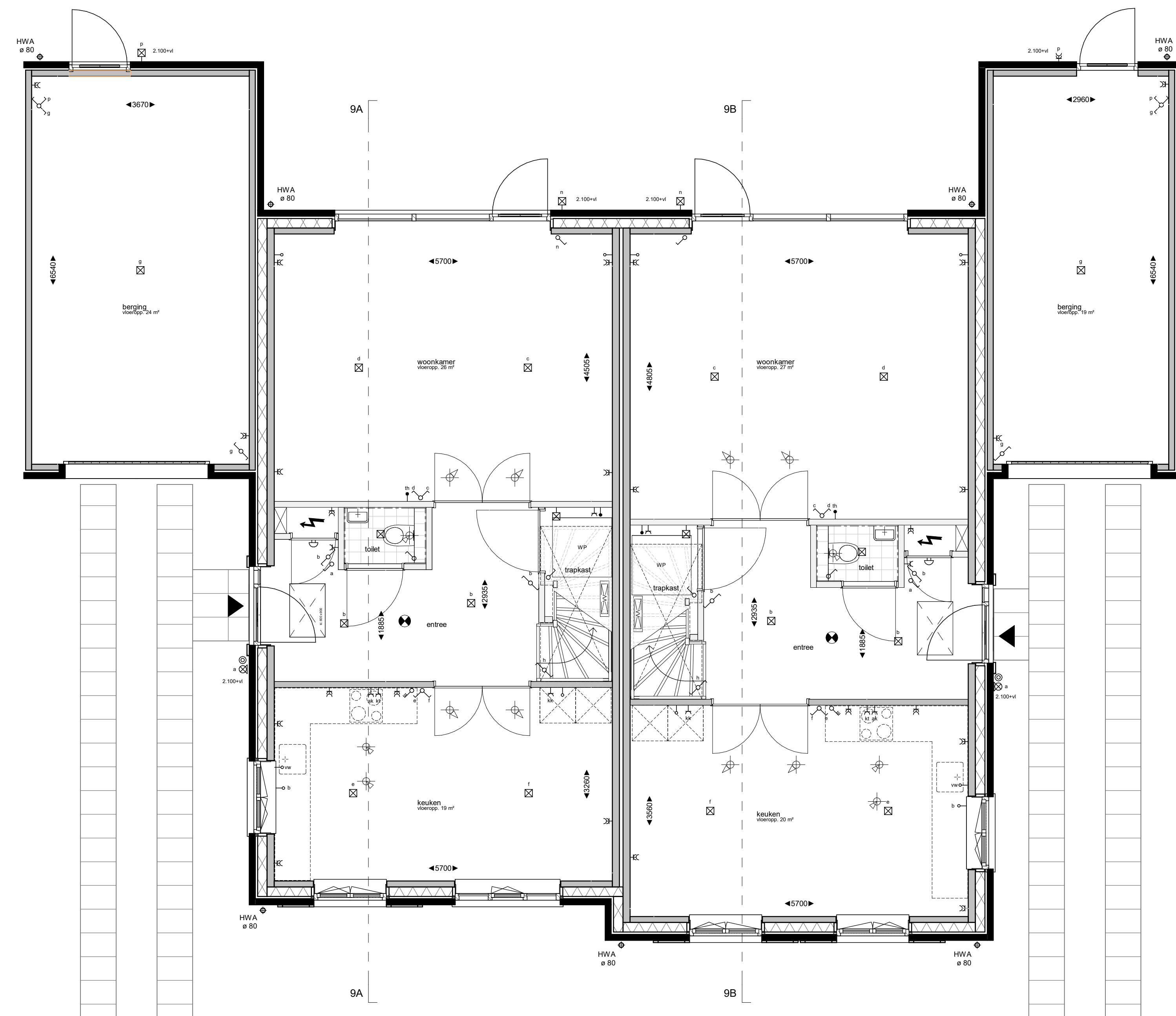
begane grond
