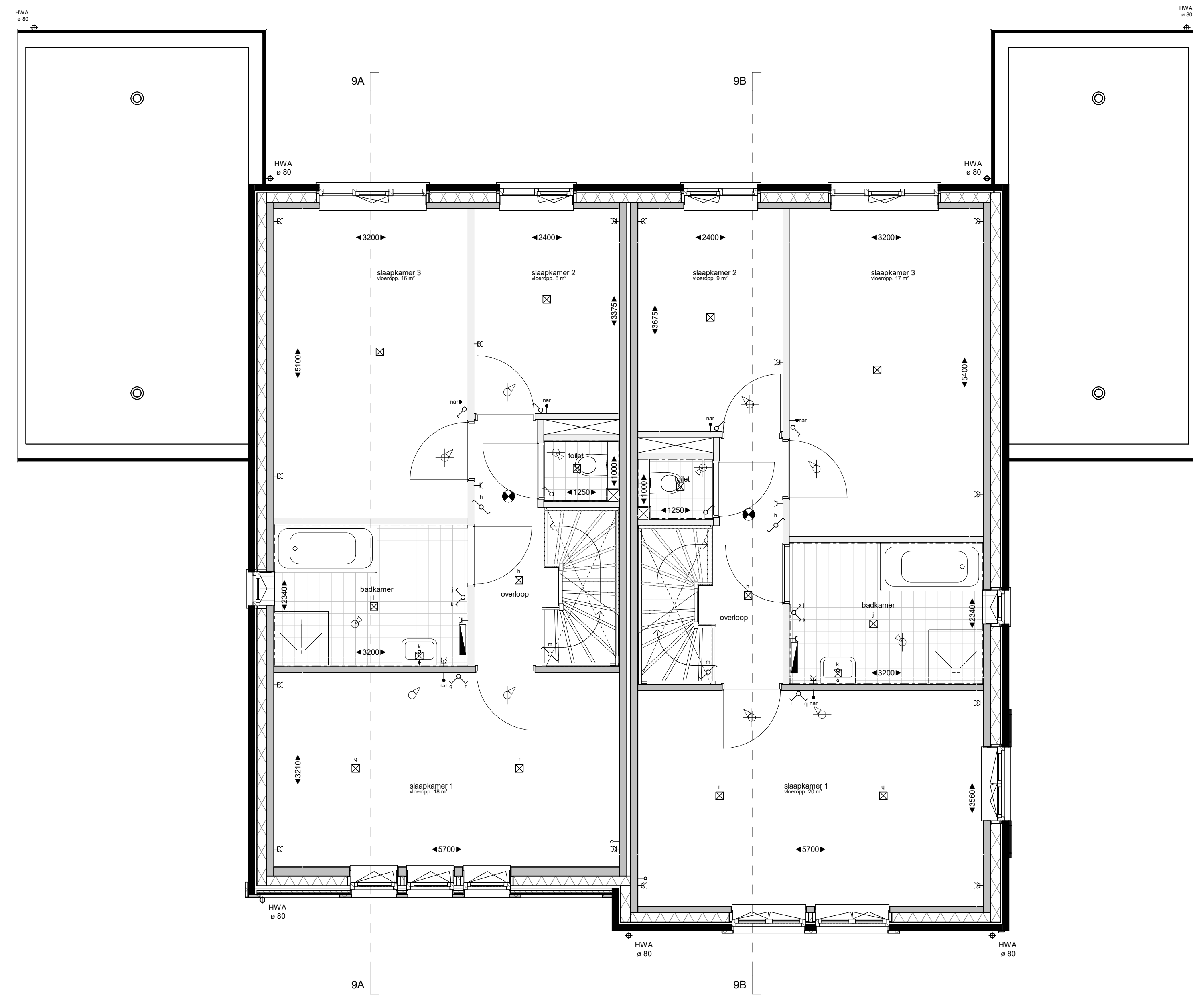
eerste verdieping
