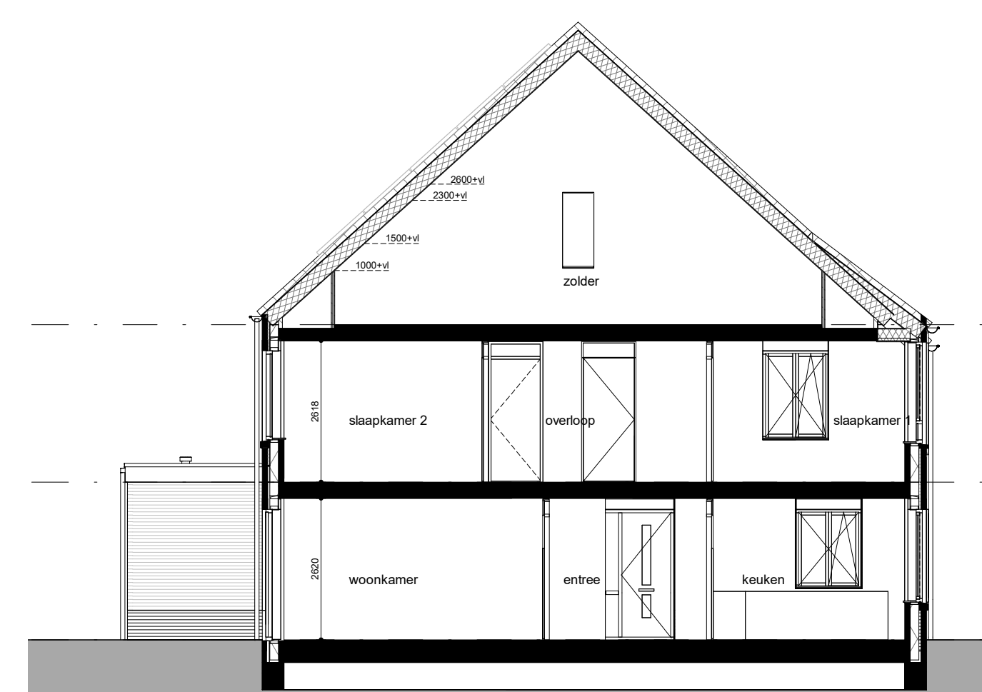
doorsnede BB
