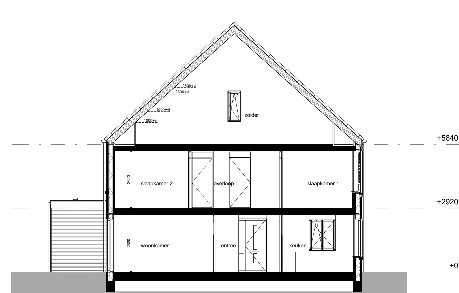
doorsnede 8B
