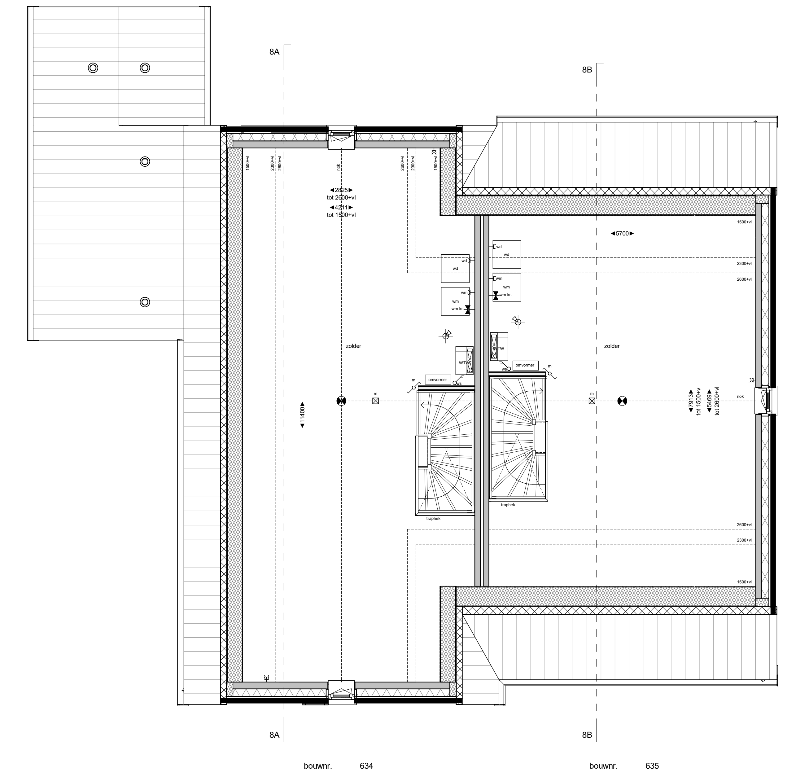
tweede verdieping
