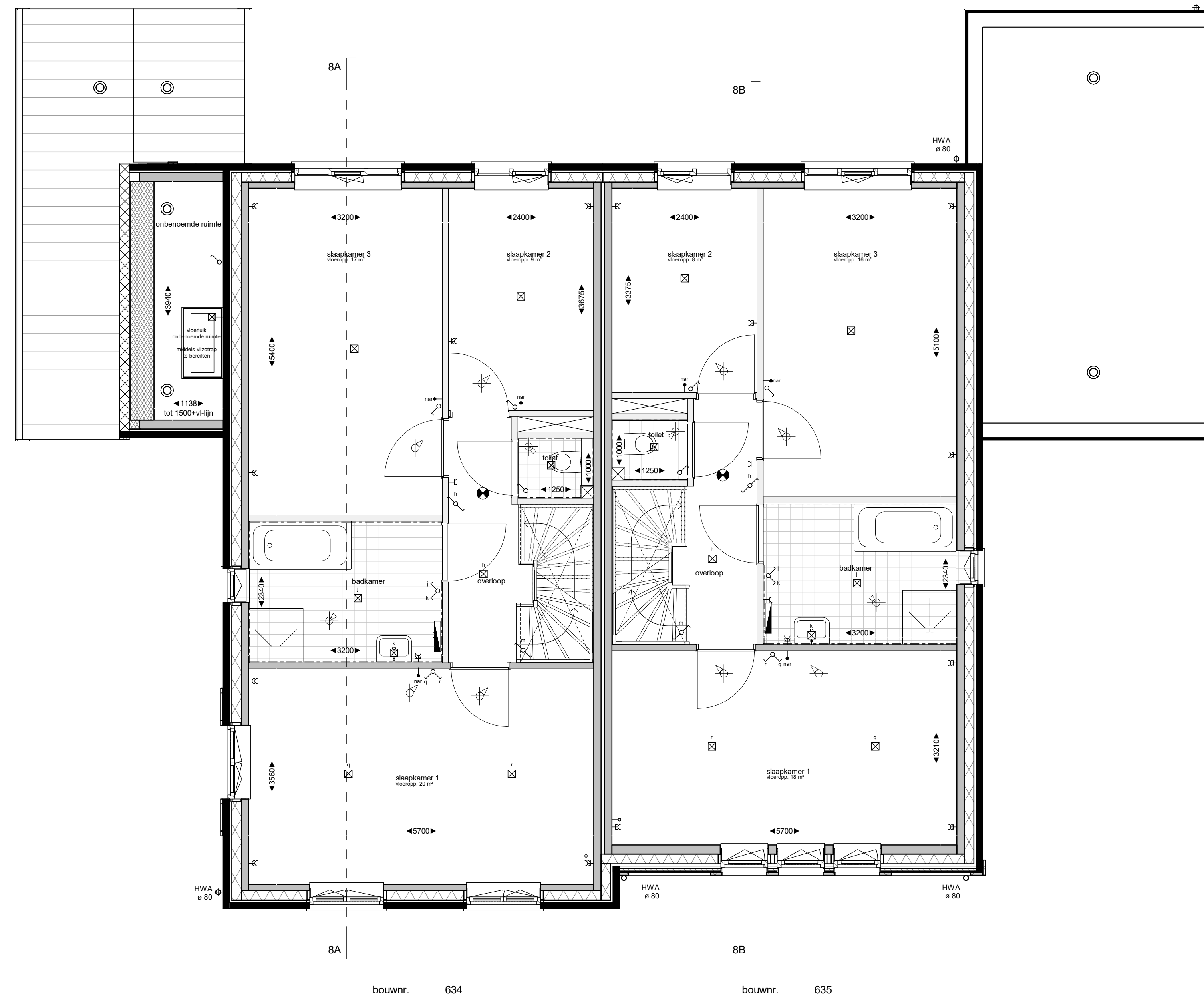
eerste verdieping
